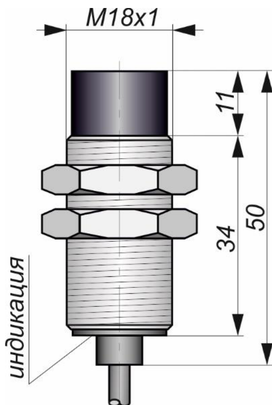
Габаритный чертеж
